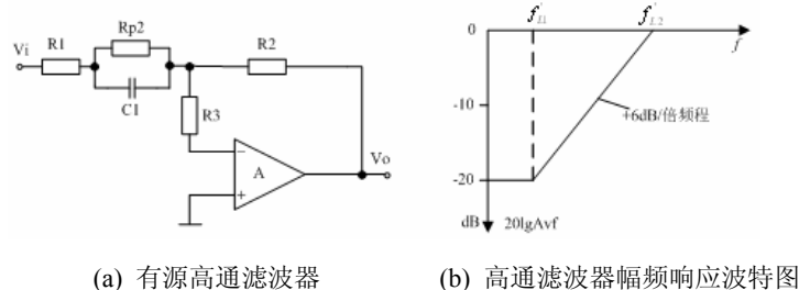
图 6.3.4 高通滤波器电路图及幅频响应曲线
