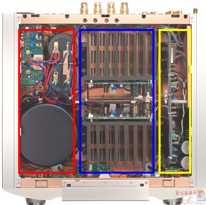
图 6.4.3 Marantz 放大机内部构造
