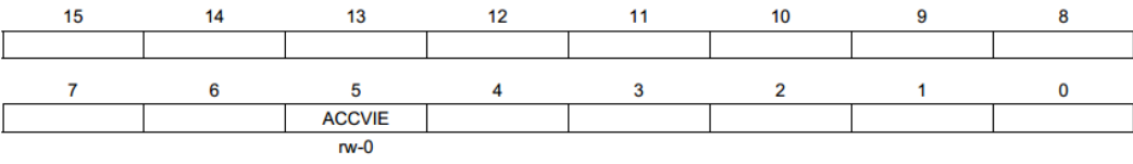
图 3.7.9 SFRIE1 寄存器
