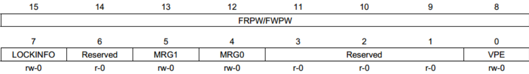
图 3.7.8 FCTL4 寄存器
