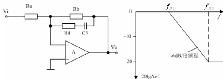
(a) 有源低通滤波器 (b) 低通滤波器幅频响应波特图
