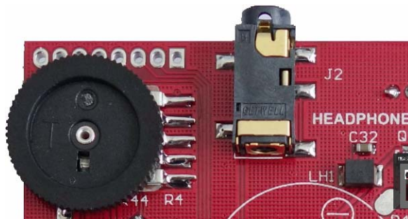
图 1.2.22 拨盘电位器模块
