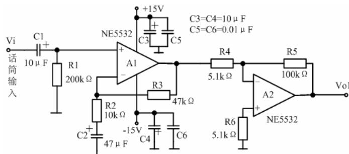
图 6.2.1 典型前置放大电路
