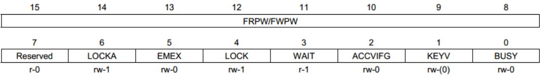
图 3.7.7 FCTL3 寄存器
