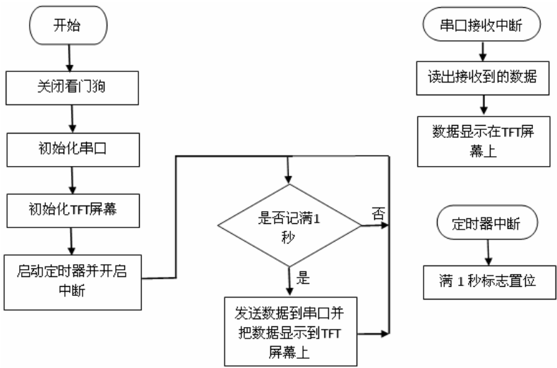
图 3.6.6 程序流程图
