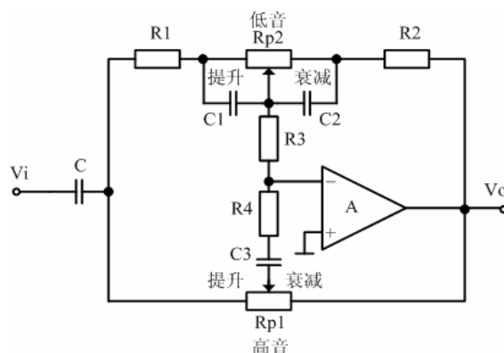
图 6.3.1 有源滤波器构成的音调控制器电路
