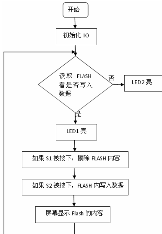
图 3.7.10 程序流程图
