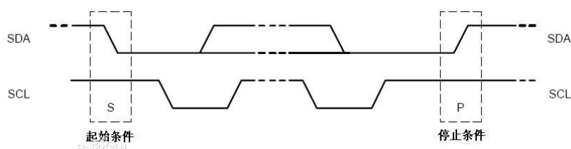
图 4.1.1 I 2 C 协议起始与终止条件
