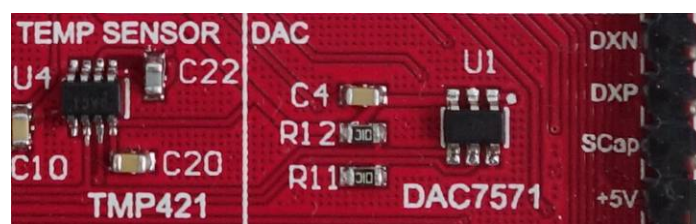
图 1.2.13 温度传感器模块
