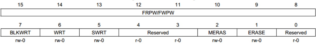
图 3.7.6 FCTL1 寄存器
