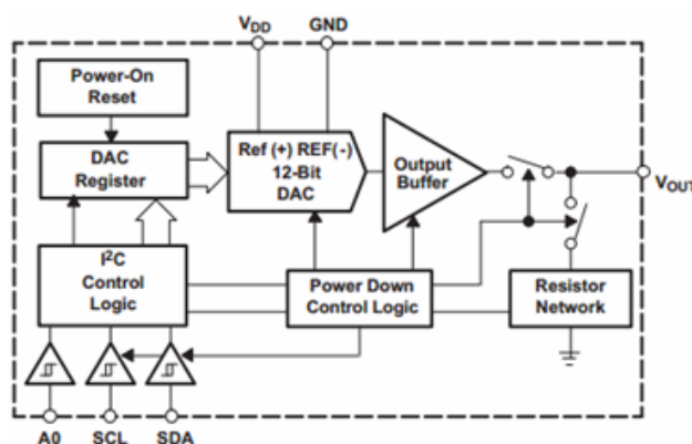
图 4.2.2 DAC7571 结构框图
